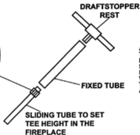
DRAFTSTOPPER INSTALLED
