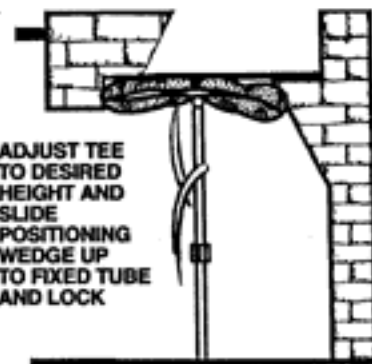
DRAFTSTOPPER INSTALLED
